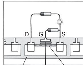
Halbleiter isolierte Ladungsschicht Stromkanal
